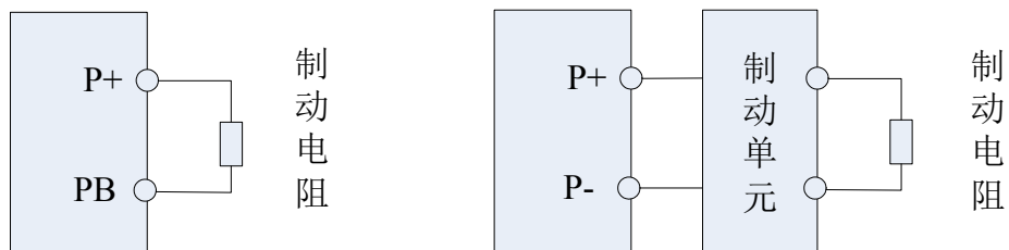
图 2-7 制动电阻连接示意图
