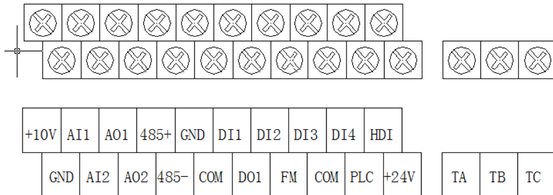
图 3-7 VL6100 控制回路端子图
