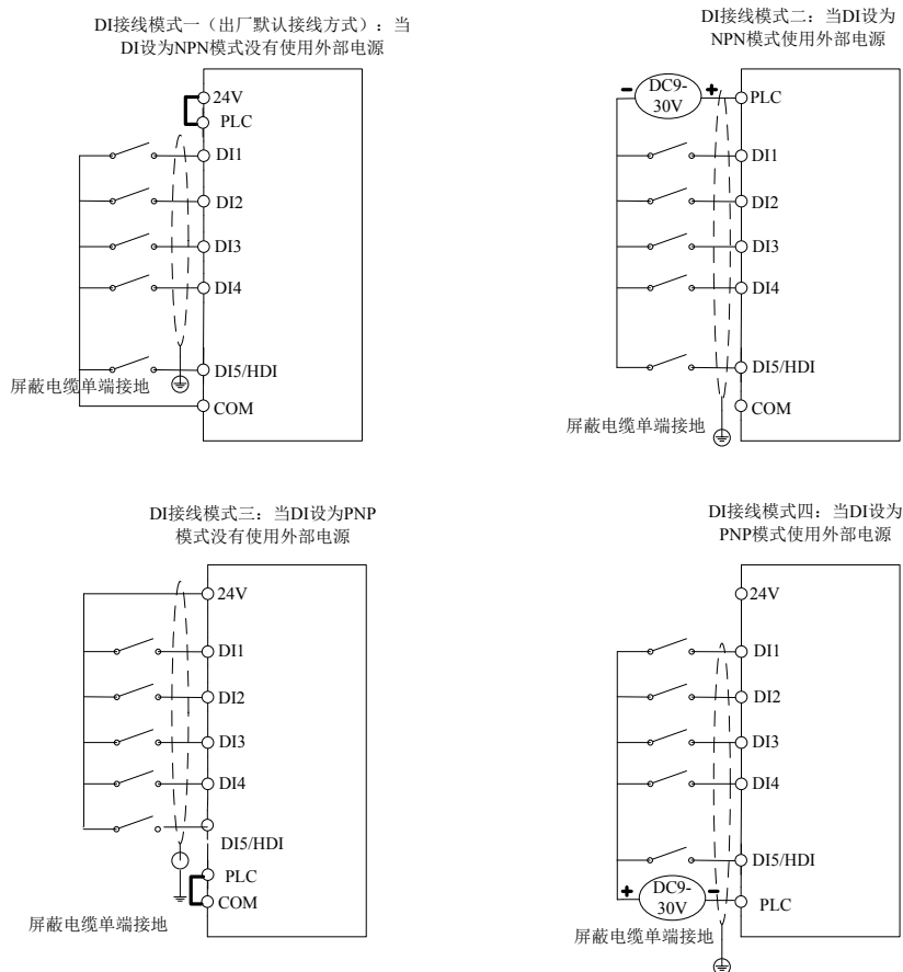
图 3-9 四种不同模式下数字输入端子接线图
