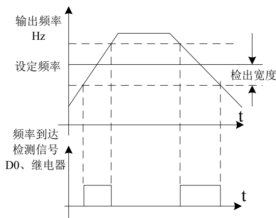
图 6-14 频率到达检出幅值示意图
