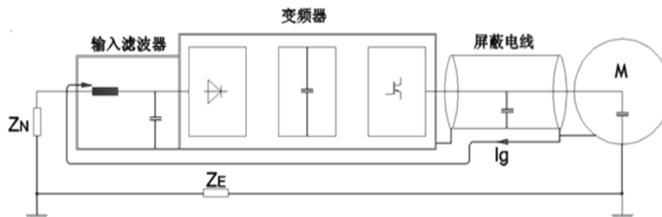
图 3-5 防传导辐射干扰接线示意图
