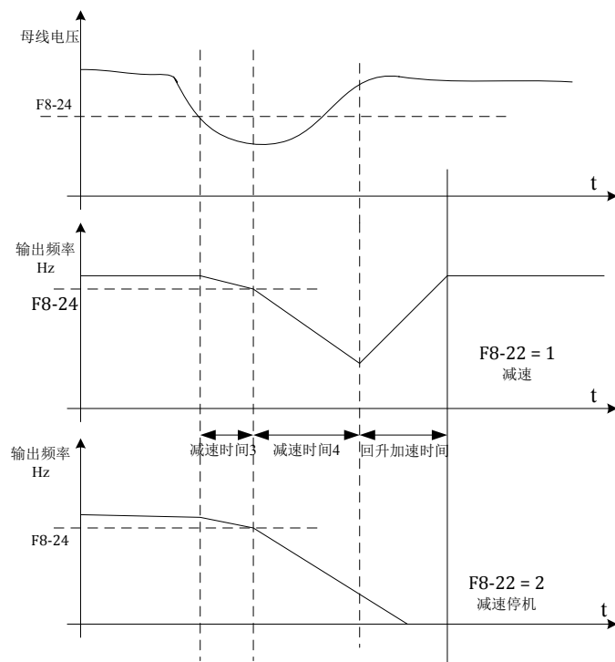
图 6-22 瞬时停电动作示意图
