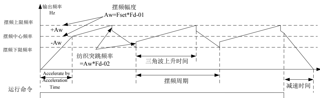
图 6-27 摆频工作示意图
