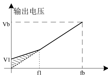
V1:手动转矩提升电压 Vb:最大输出电压 f1:手动转矩提升截止频率 fb:电机额定频率
