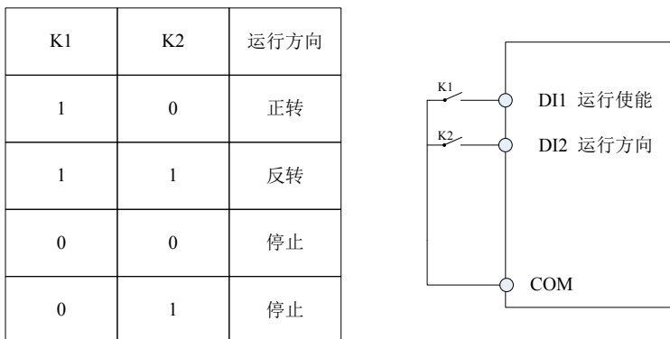
图 6-8 两线式模式 2
