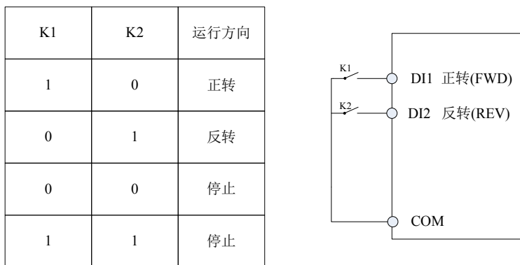
图 6-7 两线式模式 1
