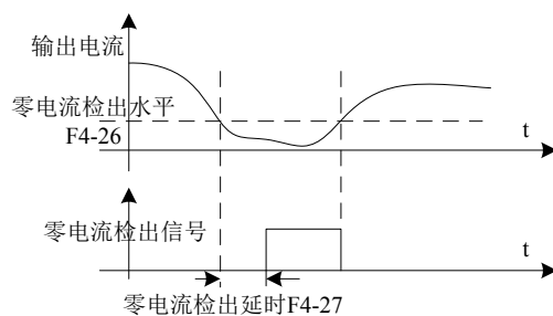
图 6-16 零电流检测示意图
