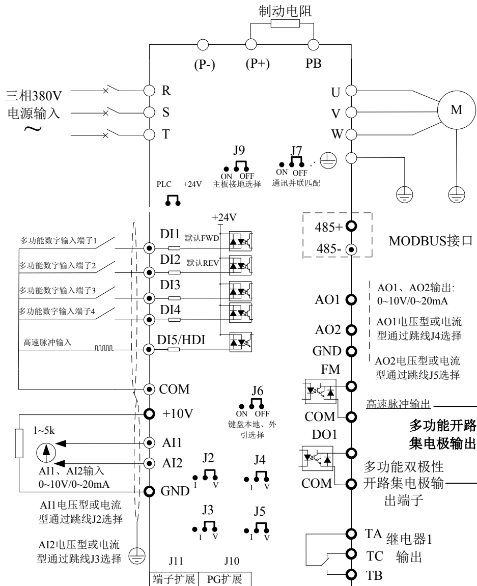
图 3-6 控制回路及主回路接线图
