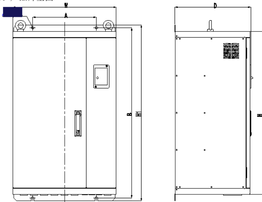
图 2-5 VL6100 系列钣金结构外型尺寸及安装尺寸示意图
