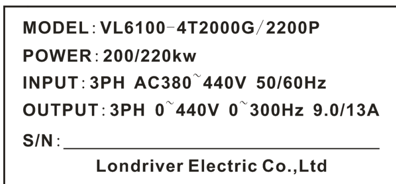
图 2-2 铭牌
