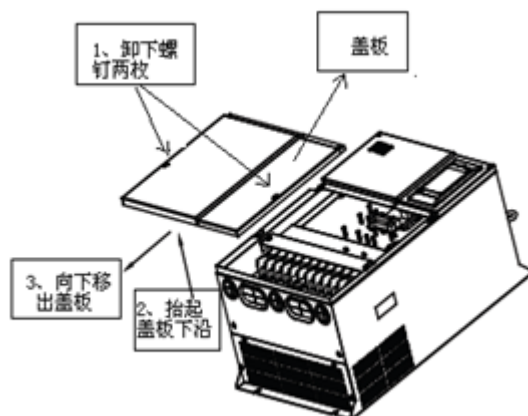
图 3-3 钣金机箱下面板的拆卸
